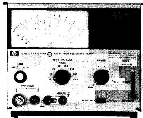
HP 4329A
